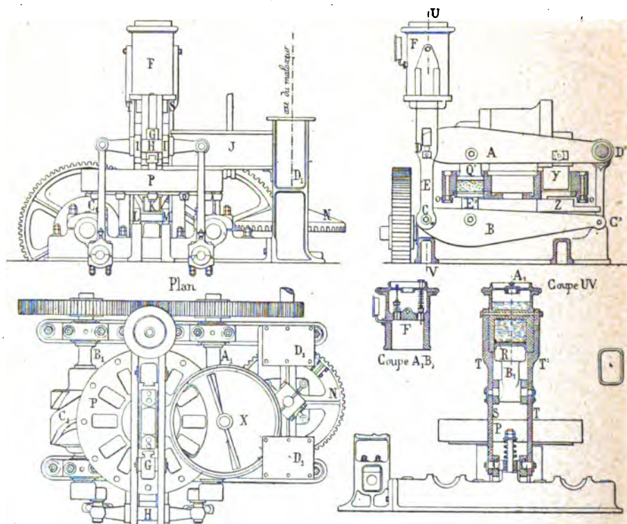
Fig. 44 à 49. — Machine Couffinhall à double compression.
